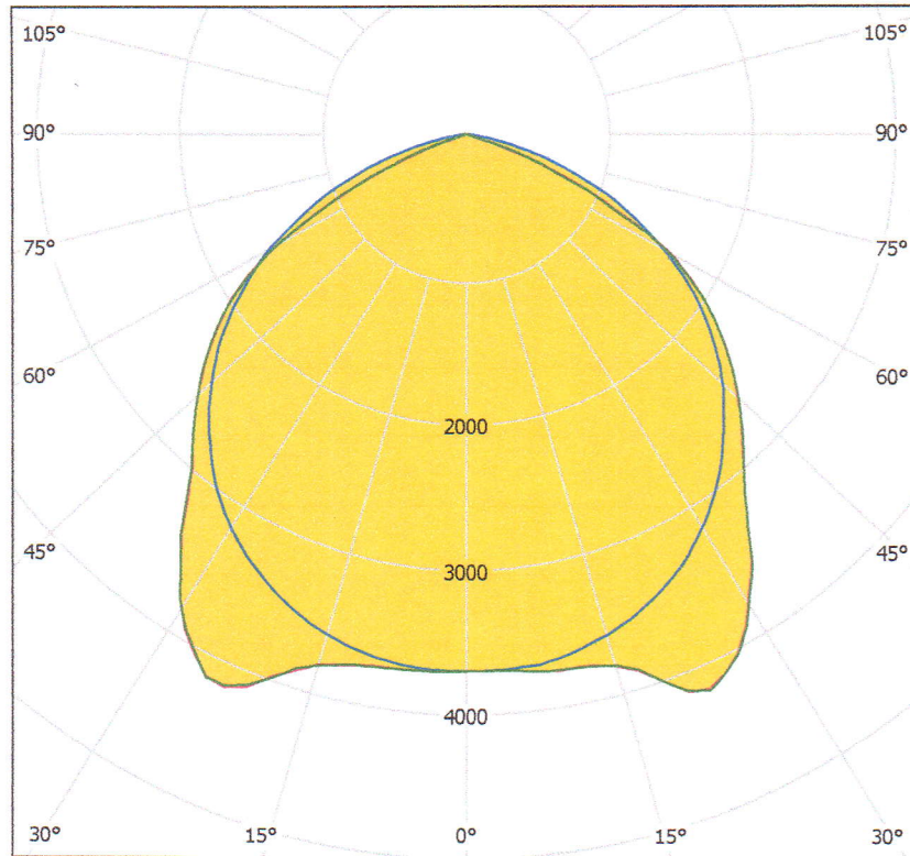
Рисунок 1 – КСС образца светильник светодиодный LuxON Promline 100W в поперечной (C0-C180) (красная кривая), продольной (C90-C270) (синяя кривая) плоскостях и плоскости максимальной силы света (C4-C184) (зеленая кривая)
