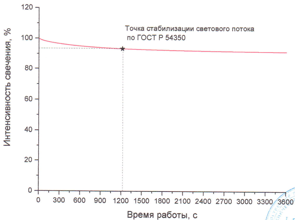
Рисунок 2 – График стабилизации светового потока образца светильник светодиодный LuxON Promline 100W
