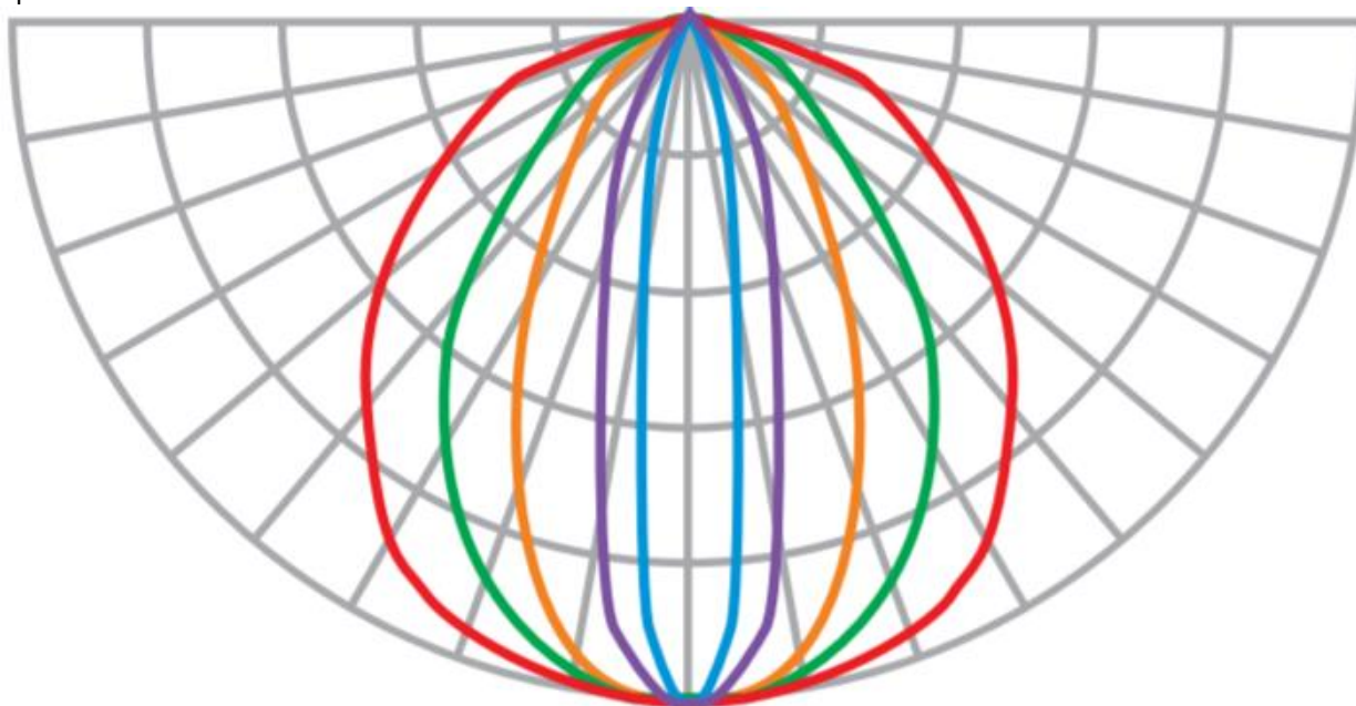
Рисунок 2. Кривые силы света для прожекторов с углом обзора 10, 25, 45, 70 и 120 соответственно
