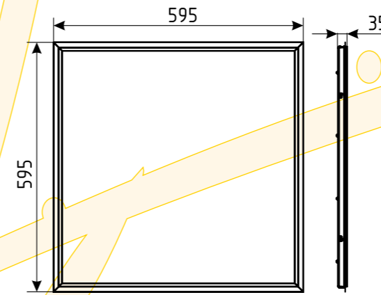
Габаритный чертеж светильника LuxON Office
