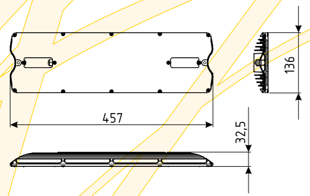
Габаритный чертеж светильника LuxON Plate
