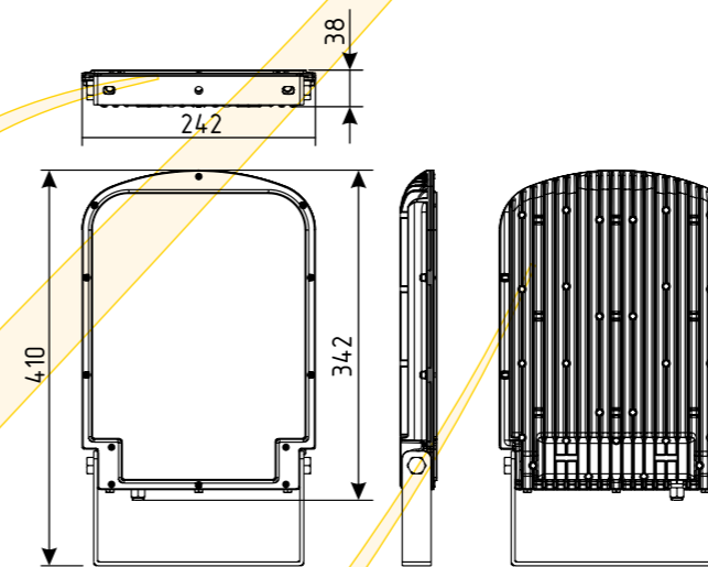
Габаритный чертеж светильника LuxON Skat
