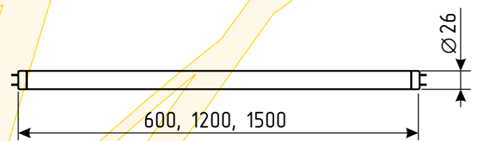
Габаритный чертеж светодиодных труб LuxON Tube
