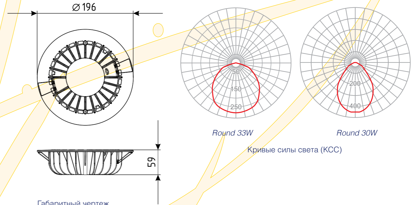
Габаритный чертеж светильника LuxON Round
