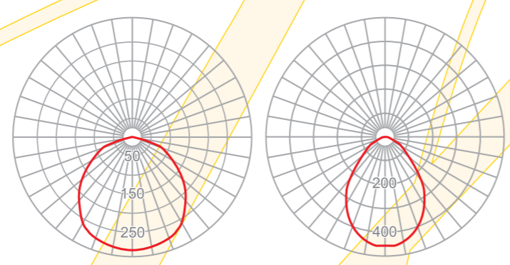
Plate 33W/44W Plate 30W Кривые силы света (КСС)
