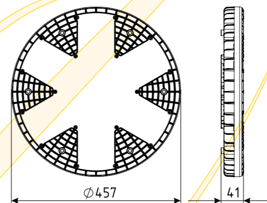
Габаритный чертеж светильника LuxON WebStar
