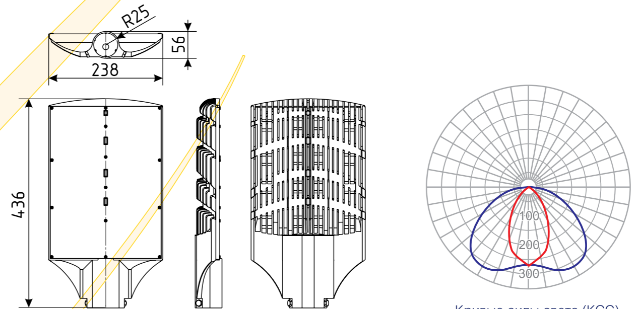
Габаритный чертеж светильника LuxON Bat
